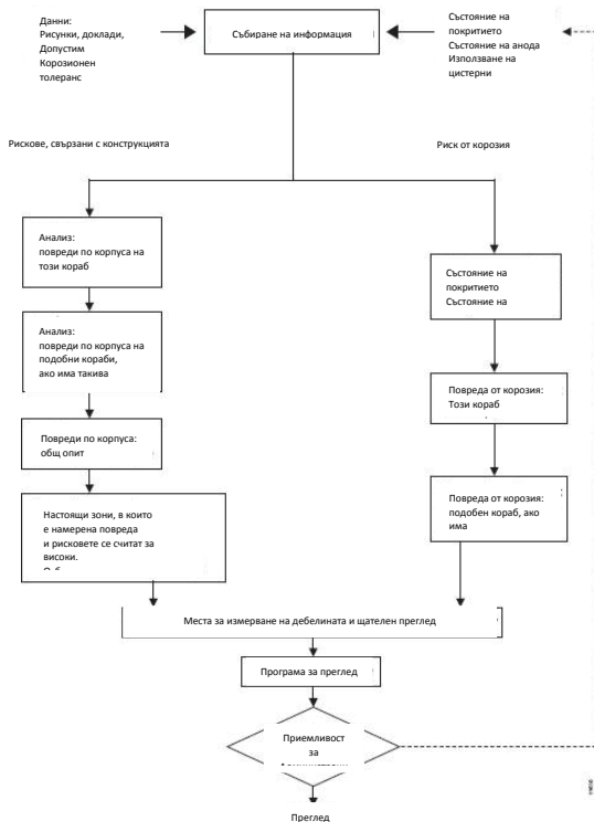
Фигура 1 - Техническа оценка и процес на планиране на преглед
