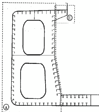
Типично напречно сечение при щателен преглед
