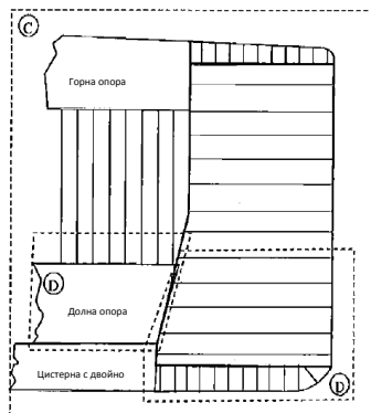
Типична напречна вертикална преграда
