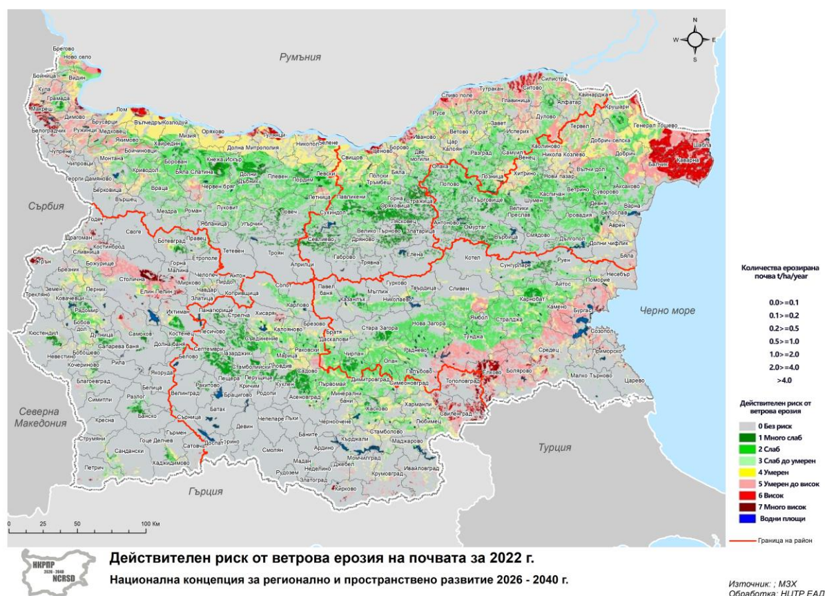
Фигура 17. Ветрова ерозия
