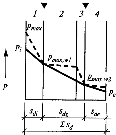
Фиг. 2.4а. Дифузия на водната пара с кондензационен пад в две равнини на оградящата конструкция или елемент (между слоеве 1 и 2 и между слоеве 3 и 4)
