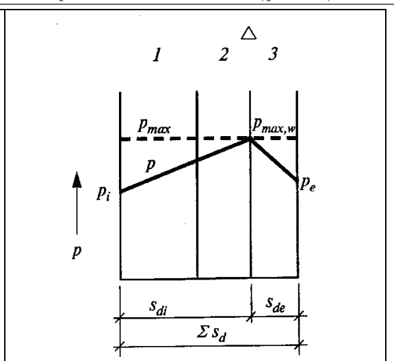
Фиг. 2.3б. Дифузия на водната пара по време на изпарението след кондензационен пад в равнината на ограждащата конструкция или елемент
