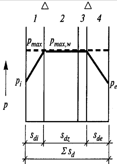
Фиг. 2.4б. Дифузия на водната пара по време на изпарението след кондензационен пад в две равнини на оградящата конструкция или елемент
